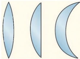
İnce Kenarlı Mercekler
