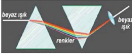
Beyaz Işığın Oluşması
