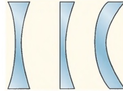
Kalın Kenarlı Mercekler
